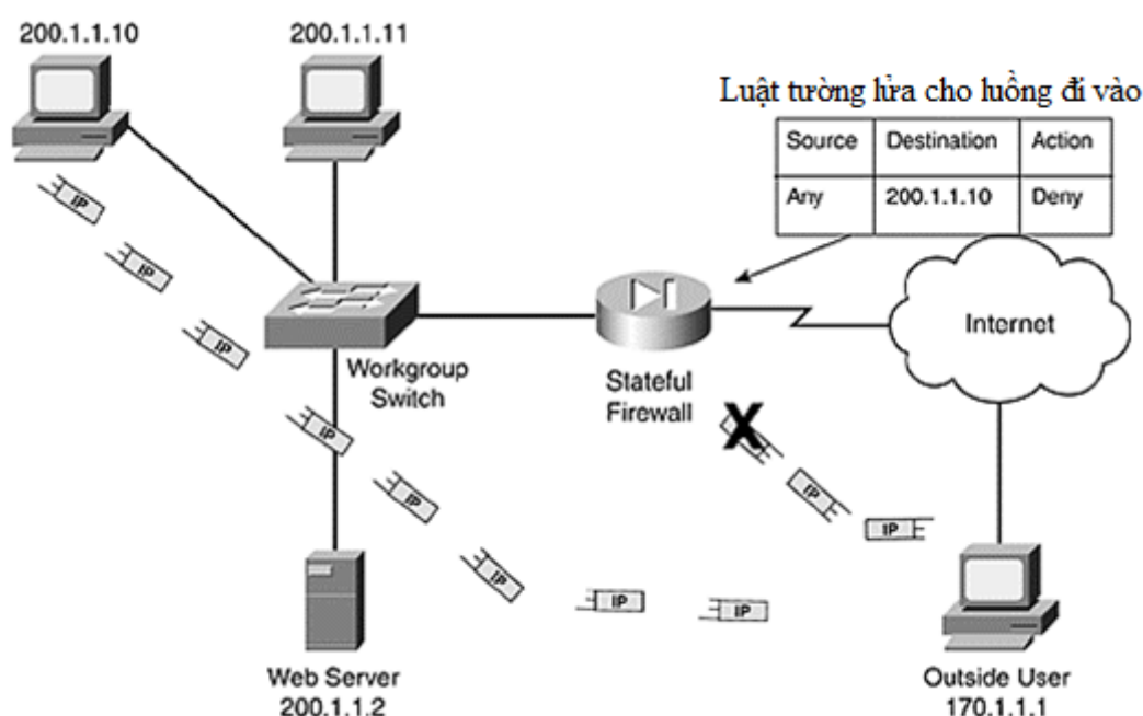
Hình 4.19. Tường lửa có trạng thái chặn gói tin không thuộc kết nối đang hoạt động
