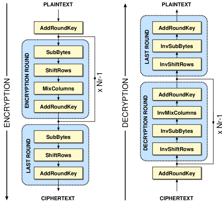
Hình 3.25. Quá trình mã hóa và giải mã trong AES
