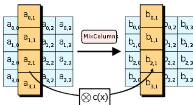
Hình 3.23. Hàm MixColumns
