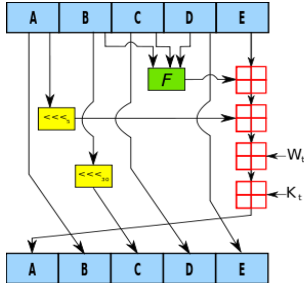
Hình 3.31. Lưu đồ một vòng xử lý của SHA1
