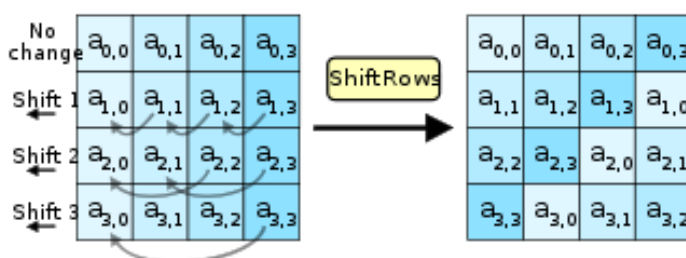
Hình 3.22. Hàm ShiftRows
