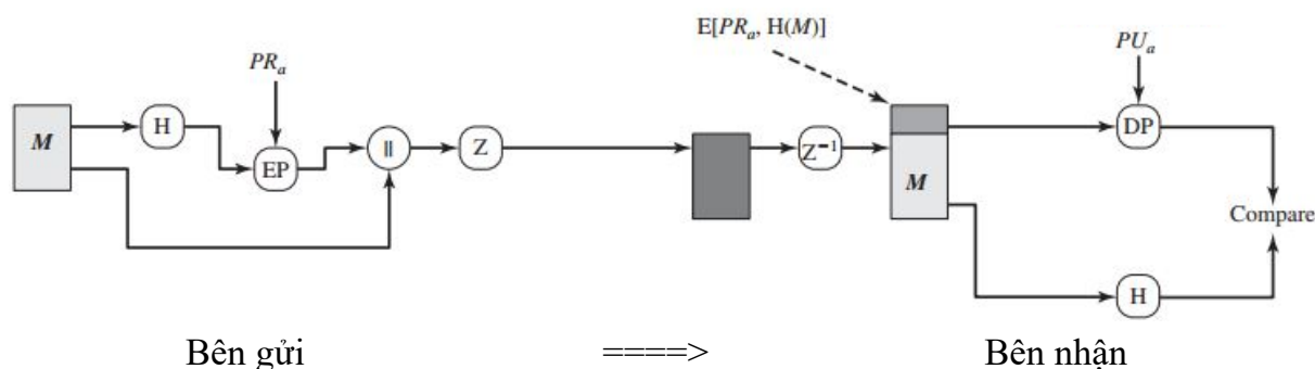
Hình 3.45. Mô hình PGP chỉ đảm bảo tính xác thực thông điệp
