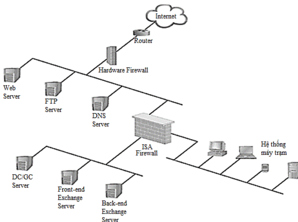
Hình 4.17. Hệ thống tường lửa bảo vệ các máy chủ dịch vụ và máy trạm
