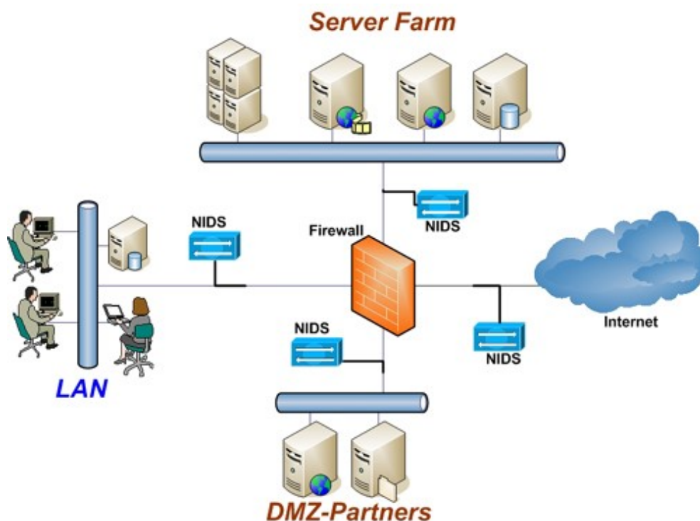
Hình 4.21. Các NIDS được bố trí để giám sát phát hiện xâm nhập tại cổng vào và cho từng phân đoạn mạng
