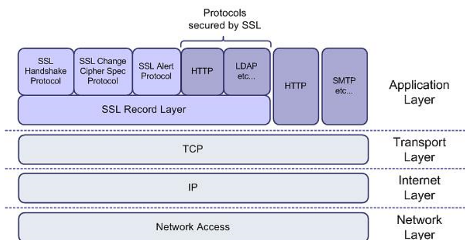
Hình 3.40. Các giao thức con của SSL/TLS
