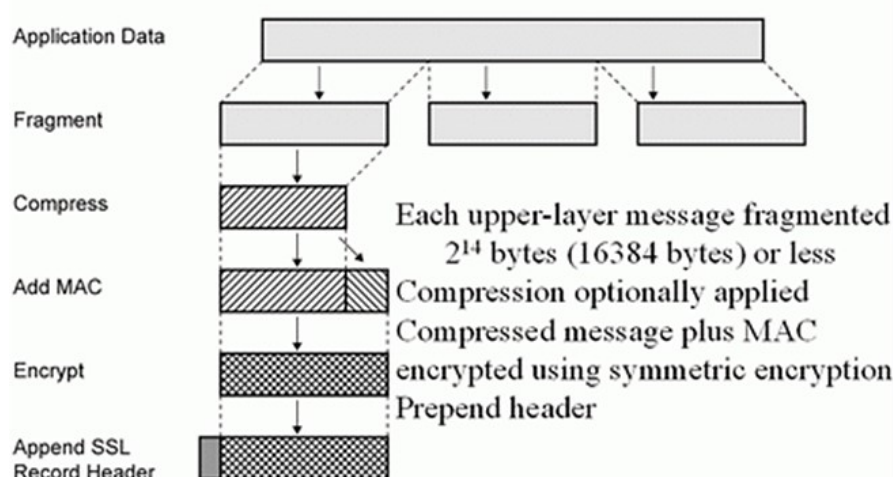
Hình 3.43. Quá trình xử lý dữ liệu bởi SSL Record tại bên gửi
