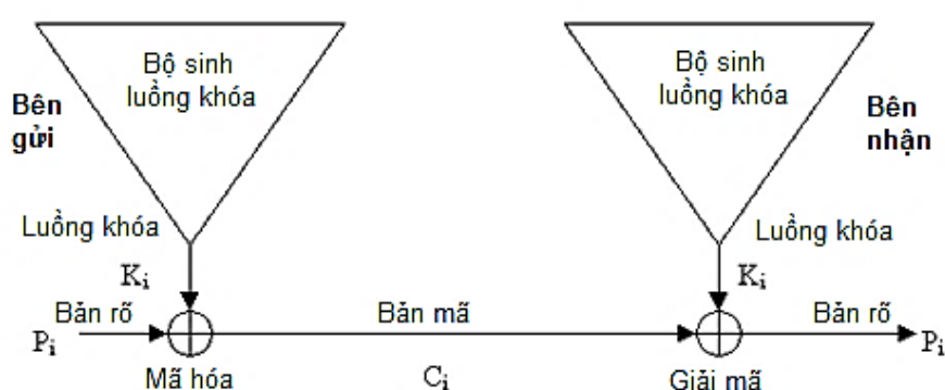
Hình 3.6. Mô hình phương pháp mã hóa dòng
