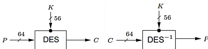
Hình 3.14. Các khâu mã hóa và giải mã của DES
