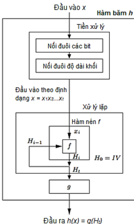
Hình 3.29. Mô hình chi tiết xử lý dữ liệu của hàm băm
