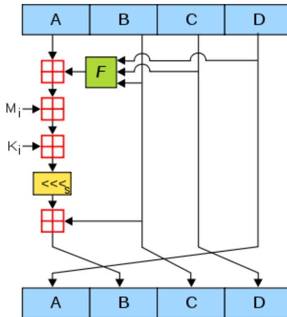
Hình 3.30. Lưu đồ xử lý một thao tác của MD5
