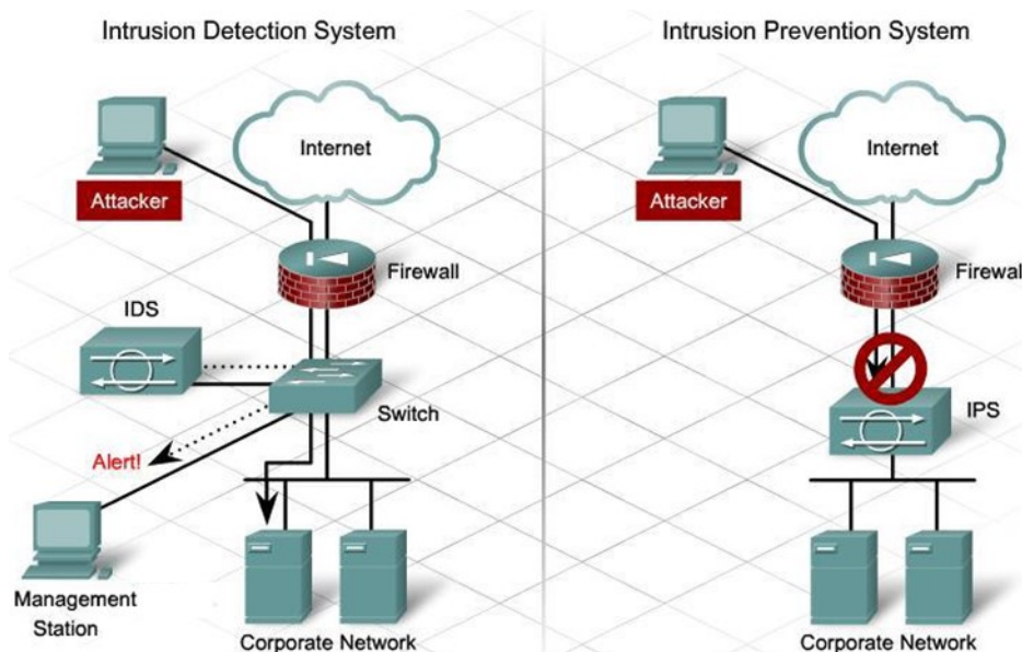
Hình 4.20. Vị trí các hệ thống IDS và IPS trong sơ đồ mạng
