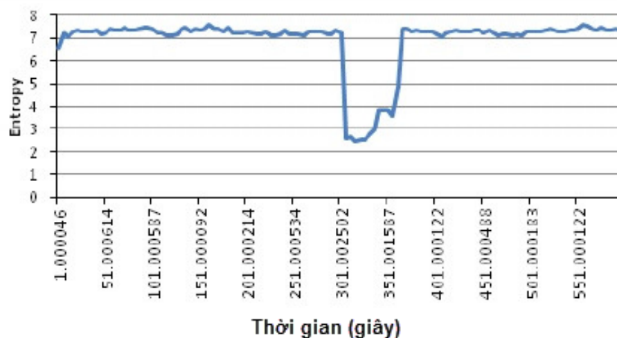
Hình 4.24. Giá trị entropy của IP nguồn của các gói tin từ lưu lượng hợp pháp (phần giá trị cao, đều) và entropy của IP nguồn của các gói tin từ lưu lượng tấn công DDoS (phần giá trị thấp)
