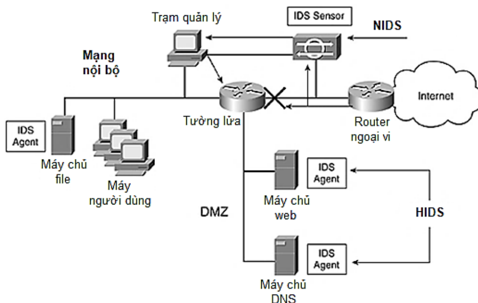
Hình 4.22. Sử dụng kết hợp NIDS và HIDS để giám sát lưu lượng mạng và các host
