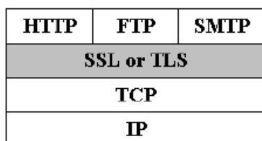
Hình 3.39. SSL/TLS trong bộ giao thức TCP/IP
