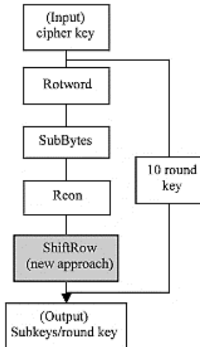
Hình 3.20. Thủ tục sinh khóa Rijndael
