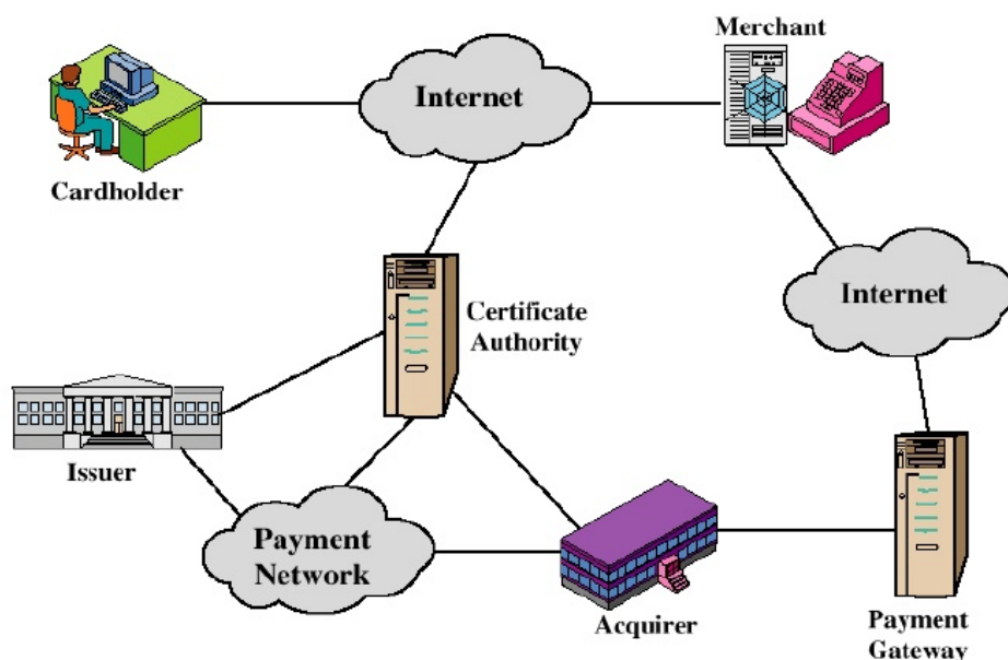
Hình 3.44. Một mô hình tương tác giữa các thực thể tham gia SET
