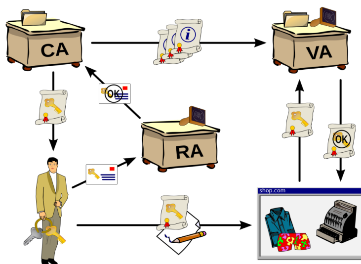
Hình 3.35. Lưu đồ cấp và sử dụng chứng chỉ số trong PKI
