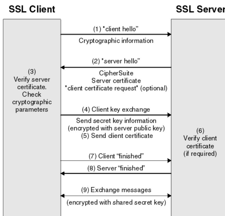
Hình 3.42. Khởi tạo phiên làm việc trong SSL/TLS
