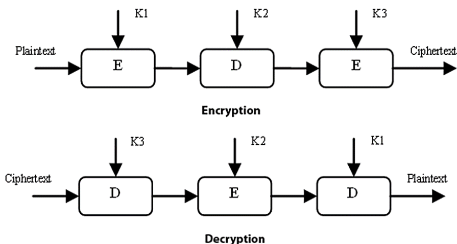
Hình 3.18. Mã hóa và giải mã với giải thuật 3-DES
