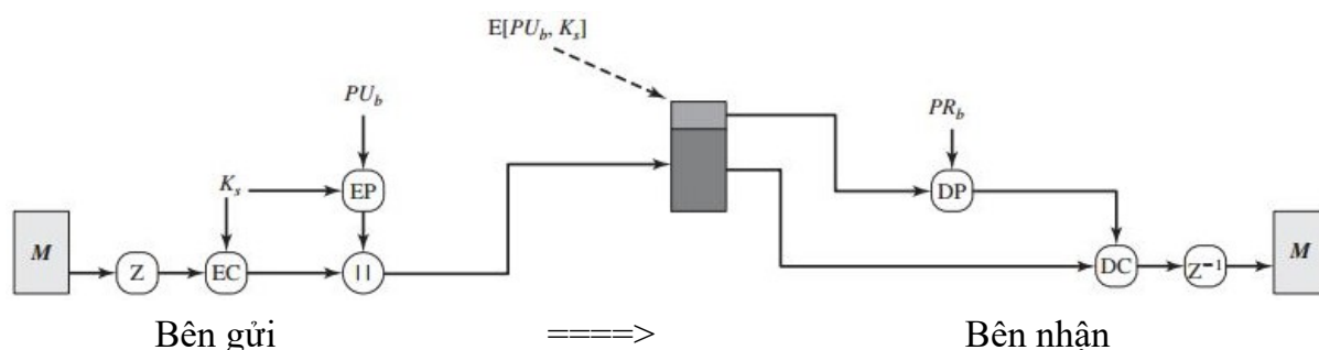
Hình 3.46. Mô hình PGP chỉ đảm bảo tính bí mật thông điệp
