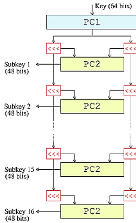
Hình 3.15. Thủ tục sinh các khóa phụ từ khóa chính của DES
