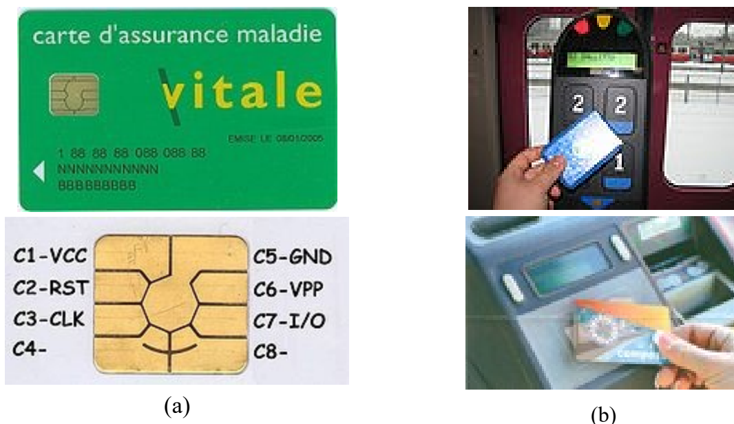
Hình 4.8. Thẻ thông minh tiếp xúc (a) và thẻ không tiếp xúc (b)
