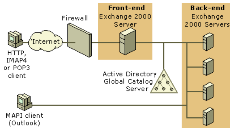
Hình 4.16. Tường lửa bảo vệ các máy chủ dịch vụ
