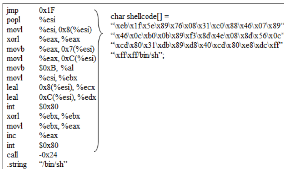
Hình 2.14. Một shellcode viết bằng hợp ngữ và chuyển thành chuỗi tấn công
