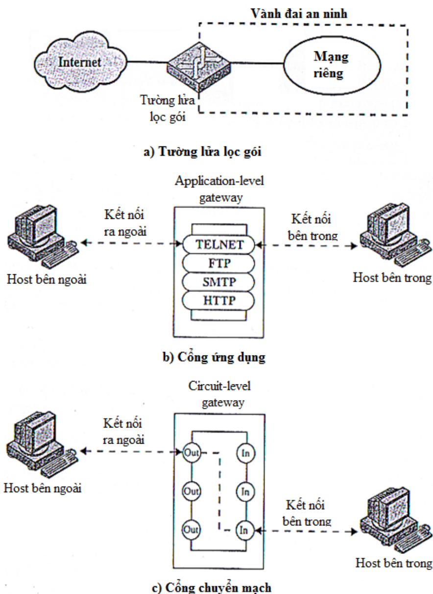
Hình 4.18. Mô hình tường lửa lọc gói (a), Cổng ứng dụng (b) và Cổng chuyển mạch (c)
